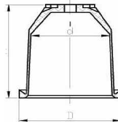
F - Clopot Ø 6 x Ø 53 x 59 cod - CL 4
