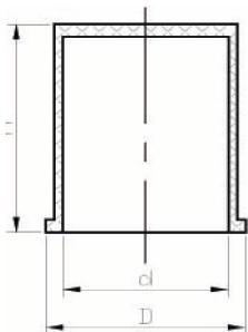
C - Clopot Ø 34 x Ø 46 x 49 cod - CL 2
