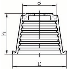
A - Clopot romex Ø 9 x Ø 52 x 46 cod - CL 3-1
